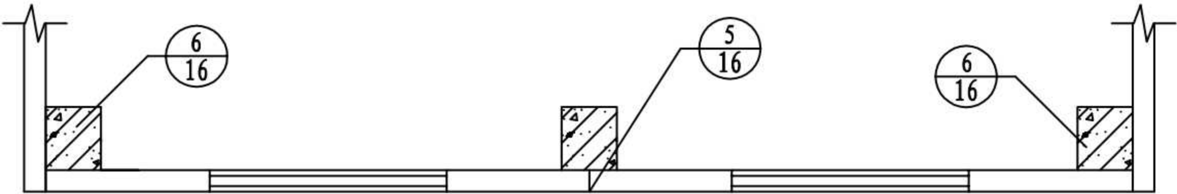
混凝土结构平面示意图(适用于外挂情况)
