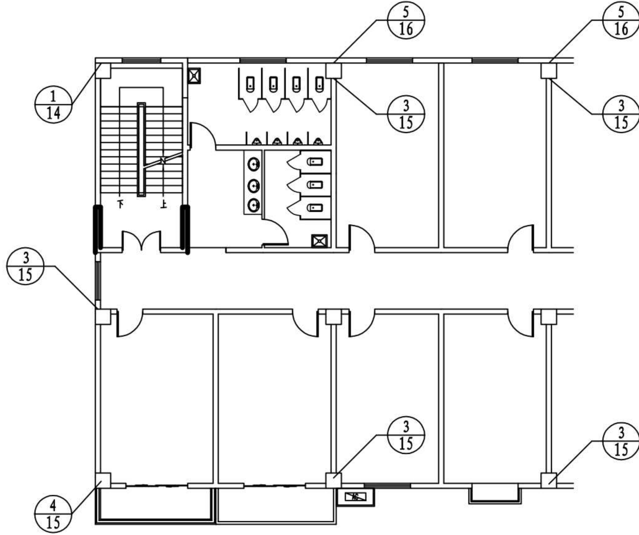
钢板网构墙板与混凝土结构连接平面示意图
