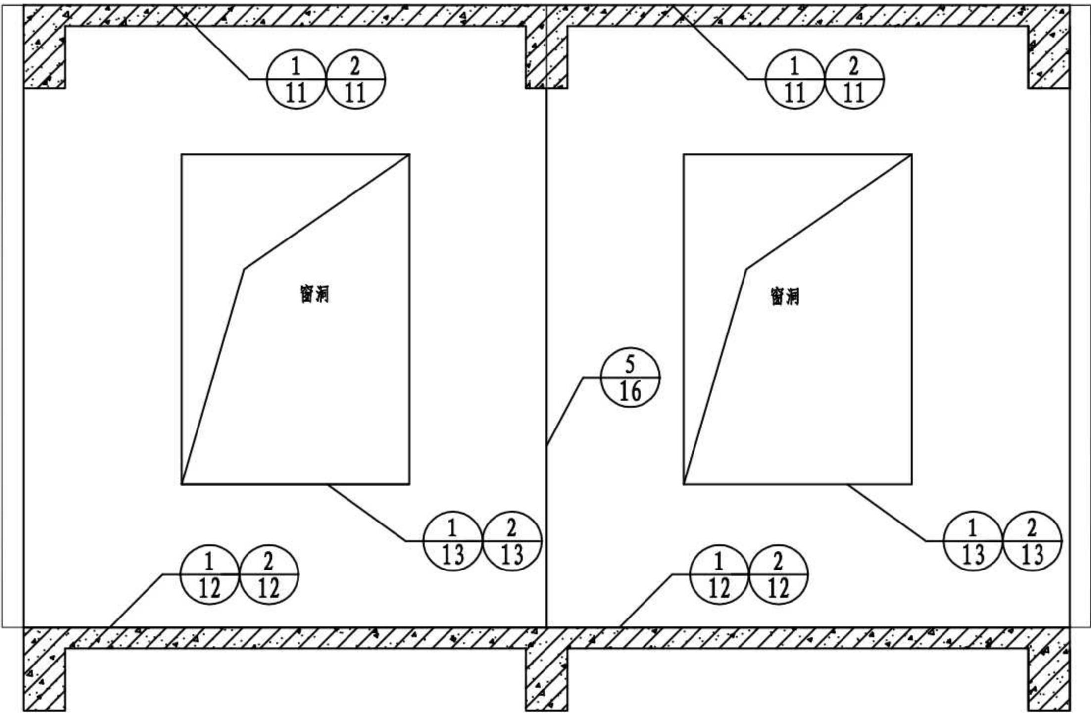
混凝土结构立面示意图(适用于外挂情况)
