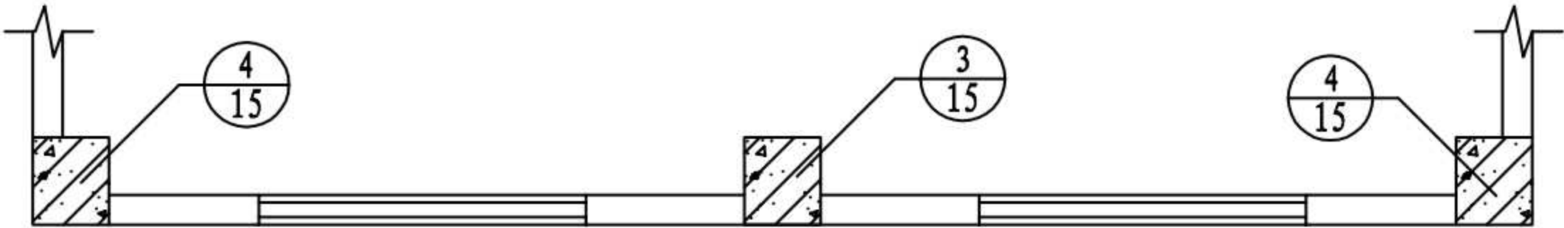
混凝土结构立面示意图(适用于内嵌情况)
