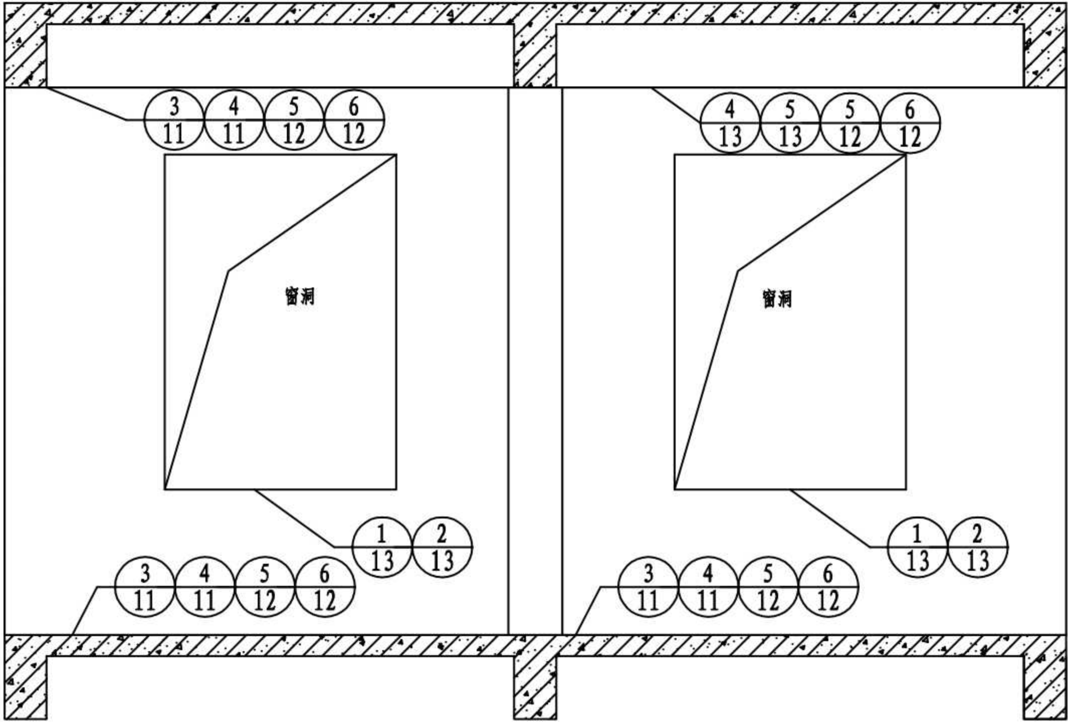
混凝土结构立面示意图(适用于内嵌情况)
