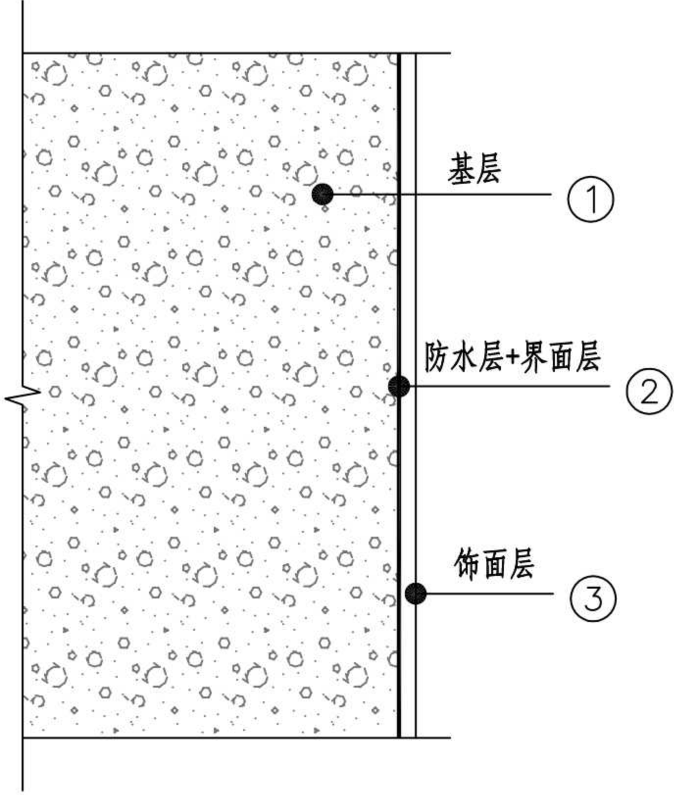
① 外墙自保温系统基本构造示意图
